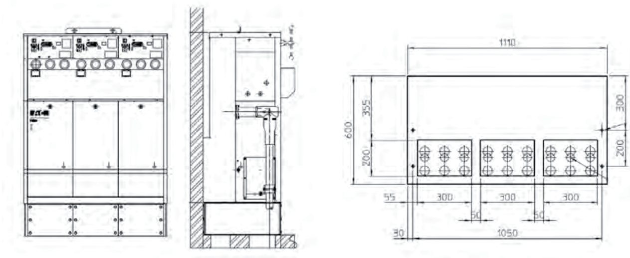
↓ Afbeelding 8. EATON Xiria KKV(m).
