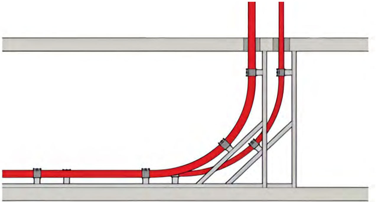
↓ Afbeelding 5. kelder met kabelopvoerconstructie.
