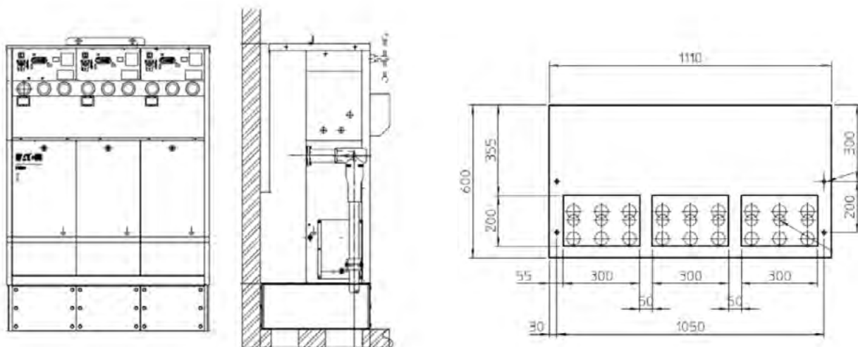
↓ Afbeelding 8. Eaton Xiria KKV(m).
